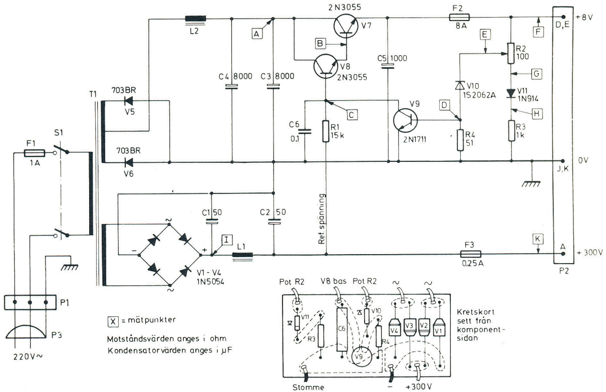
Kretsschema
