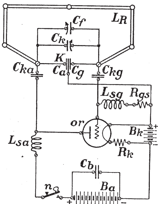
Fig. 10. Förenklat kopplingschema för sändaren.
