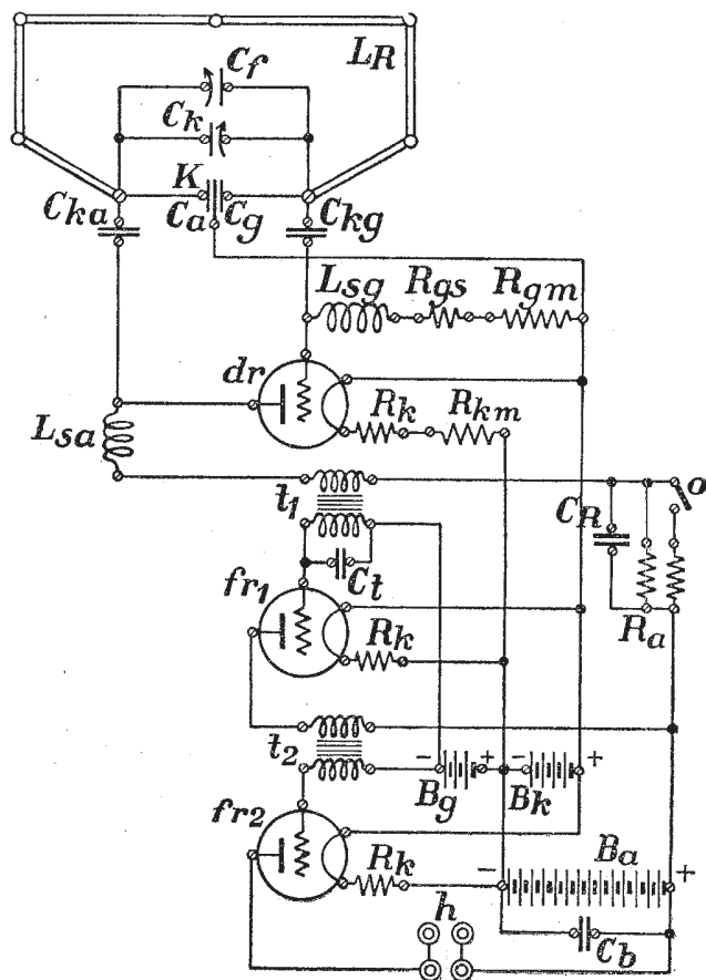
Fig. 9. Förenklat kopplingsschema för mottagaren.
