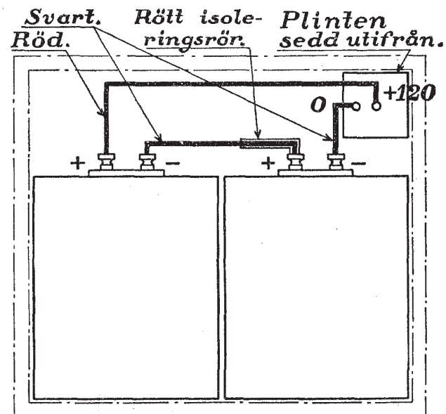
Fig. 6. Kopplingsschema över batterilådan.
