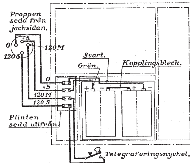
Fig. 4. Kopplingsschema över materiellådan.
