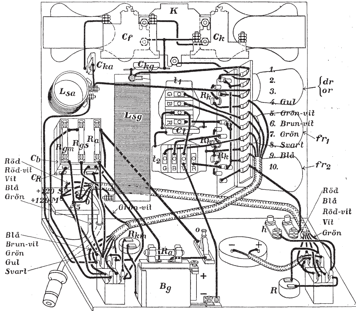
Perspektivschema för apparaten.
