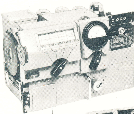
Sändarenhet
