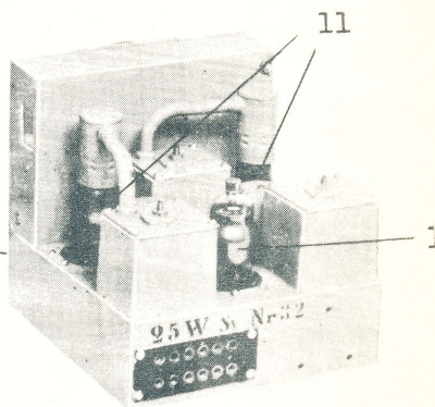
7 Mottagarenhet B-del
