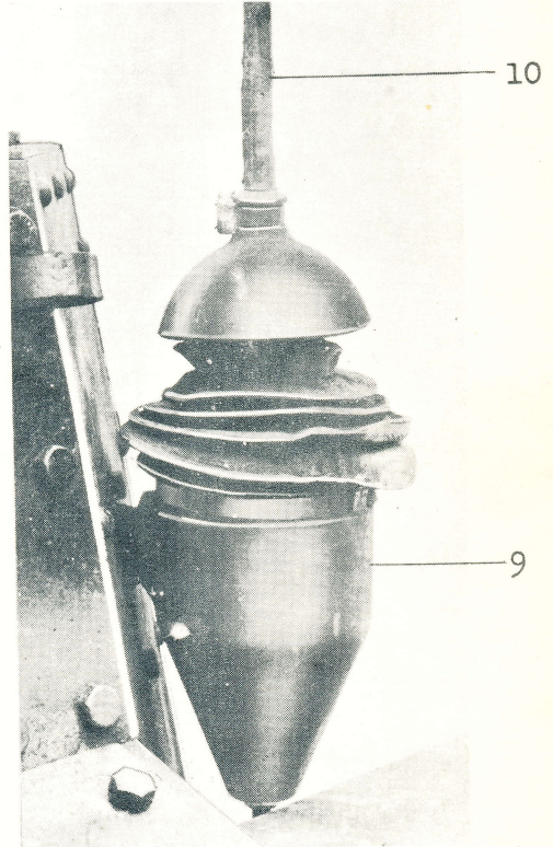
Anordningar inuti stridsvagnen för antennens upp- och nedfällning.
