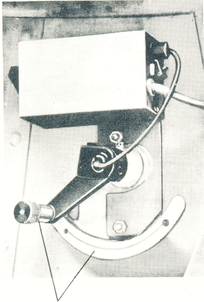
Anordningar inuti stridsvagnen för antennens upp- och nedfällning.
